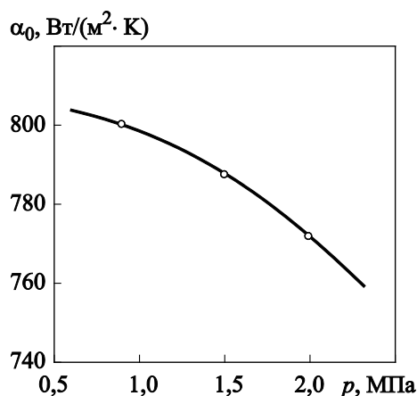
Рис. 11. Экспериментальный график зависимости коэффициента теплоотдачи \alpha_0 от давления p для масла марки МС-20. Экспериментальные значения \alpha_0 (о)
