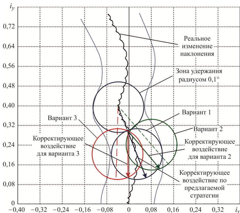
Рис. 6. Графическое отображение предлагаемой стратегии коррекции наклонения для радиусов удержания менее 0,2^\circ
