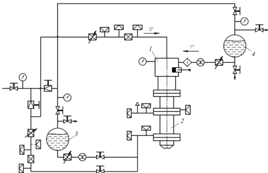
Рис. 2. ПГС стенда:
