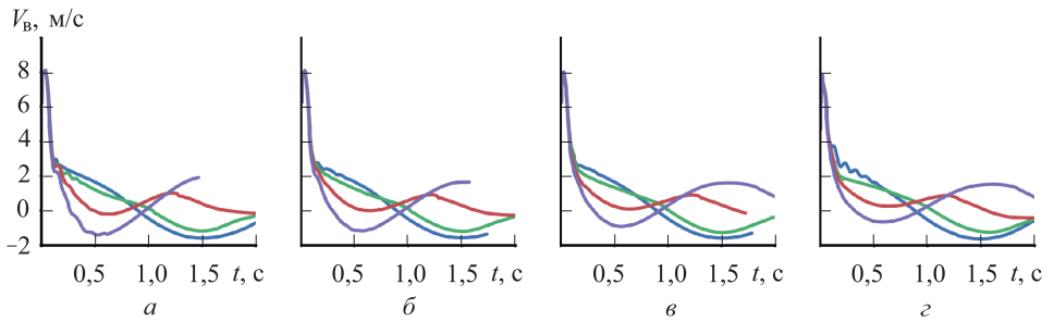
Рис. 11. Скорость центра масс в ГСК в расчетах при \varphi_\alpha = 0^\circ ( a ), \varphi_\alpha = 5^\circ ( b ), \varphi_\alpha = 10^\circ ( \bar{b} ) и \varphi_\alpha = 15^\circ ( \bar{b} ) и значениях V_r , м/с: — — 0; — — 5; — — 10; — — 15
