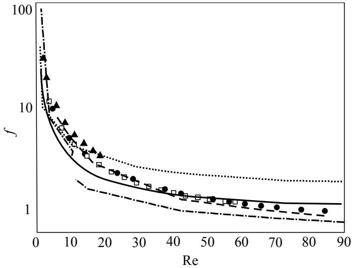
Рис. 11. Опубликованные экспериментальные данные и расчетное значение зависимости фактора трения f от числа Re :
