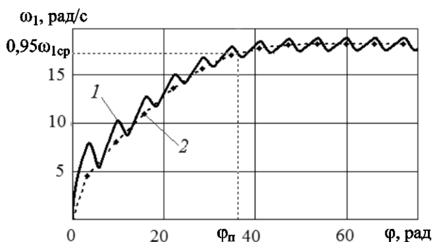
Рис. 9. Изменение угловой скорости начального звена (1) и ее средние значения за один оборот (2)
