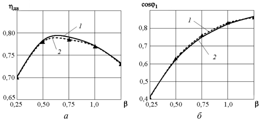
Рис. 4. Зависимость КПД (а) и коэффициента мощности (б) от коэффициента загрузки двигателя: 1 — расчетная; 2 — полученная по данным [9]
