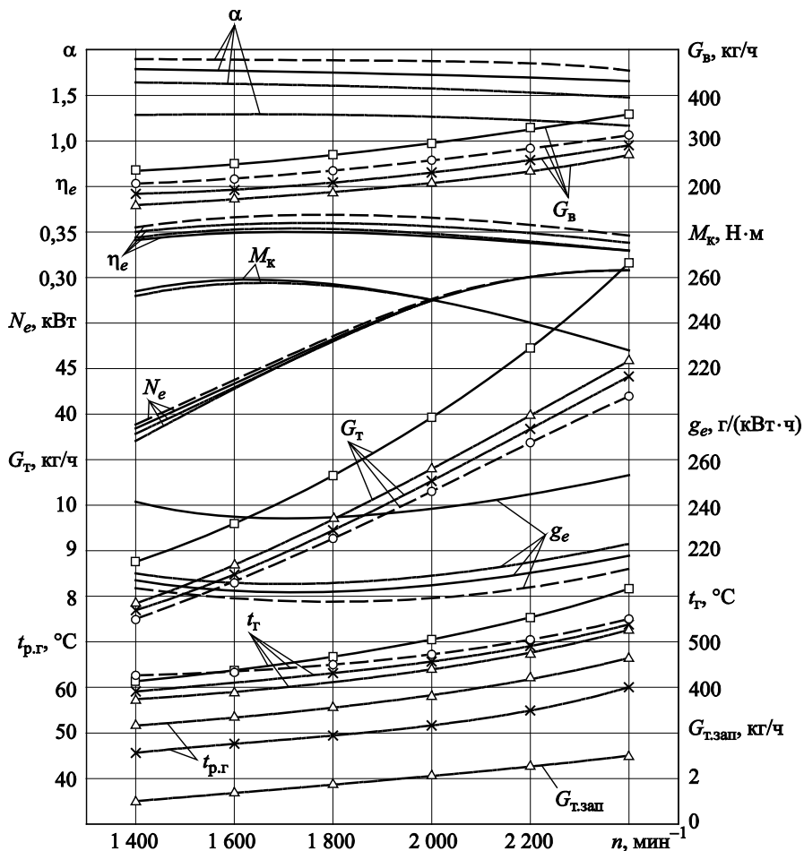
Рис. 1. Зависимость эффективных показателей работы дизеля 4С 11,0/12,5 от частоты вращения коленчатого вала без регуляторной ветви при \Theta_{\text{впр}} = 23^\circ : ■ — дизельный процесс; ○ — газодизельный процесс; × — газодизельный процесс с рециркуляцией 10 %; ▲ — газодизельный процесс с рециркуляцией 20 %; ▲ — расход запального дизельного топлива
