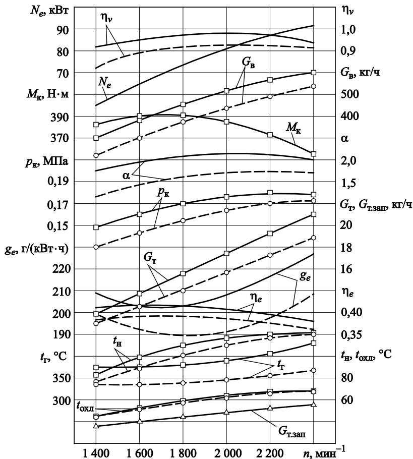
Рис. 5. Зависимость эффективных показателей дизеля 4ЧН 11,0/12,5 с охлаждением наддувочного воздуха от частоты вращения коленчатого вала: □ — N_e , — N_e — дизельный процесс; ○ — \eta_e , ○ — \eta_e — газодизельный процесс; △ — G_{t.zap} — расход запального дизельного топлива
