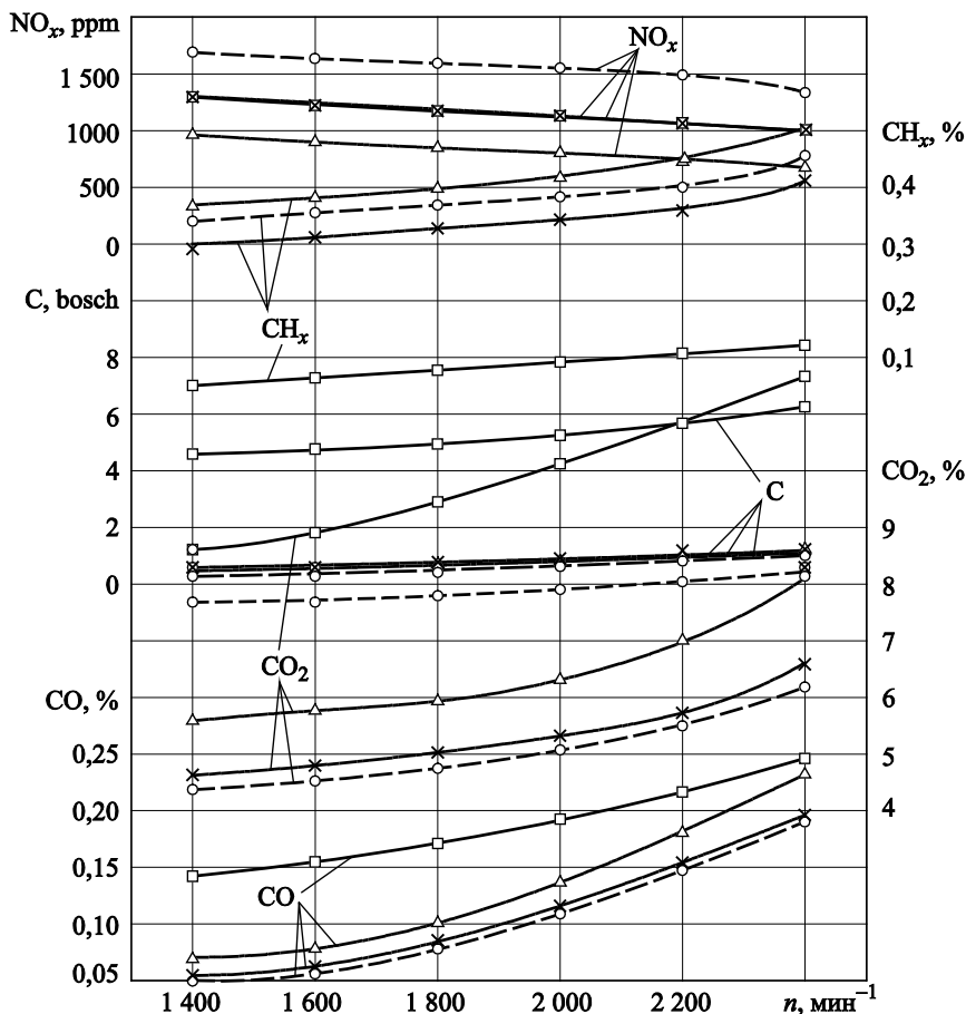
Рис. 2. Зависимости содержания токсичных компонентов в ОГ дизеля 4Ч 11,0/12,5 от частоты вращения коленчатого вала при \Theta_{впр} = 23^\circ :
