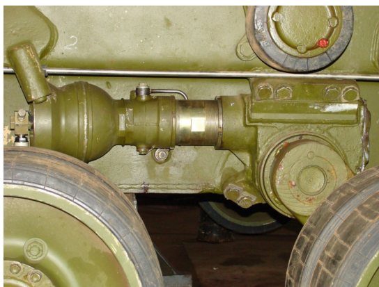
Рис. 2. Место установки ПГСП с встроенной ПГР в ходовой части гусеничной машины
