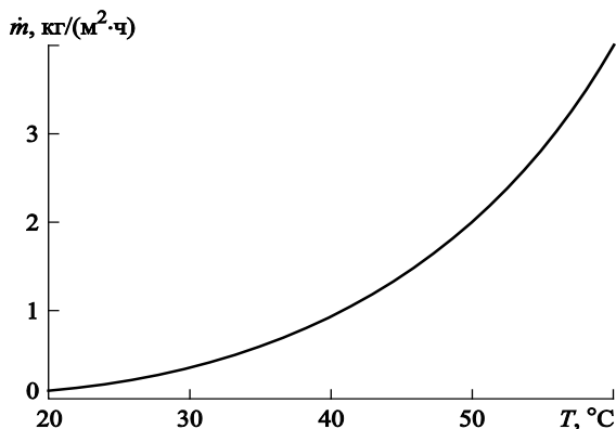
Рис. 4. Изменение плотности потока массы воды, испаряющейся с открытой поверхности, в процессе нагрева
