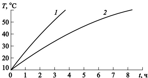
Рис. 2. Температура воды в резервуаре при относительной мощности нагрева 17 (1) и 8,5 (2) Вт/кг в зависимости от времени нагрева
