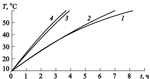
Рис. 7. Изменение температуры воды в процессе нагрева при открытой поверхности резервуара с относительной мощностью нагрева 8,5 (1) и 17 (3) Вт/кг в сравнении с нагревом при поверхности воды, закрытой полыми сферическими изоляторами, с относительной мощностью нагрева 8,5 (2) и 17 (4) Вт/кг
