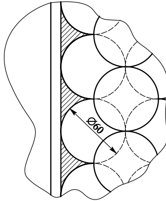
Рис. 5. Схема размещения сферических изоляторов на свободной водной поверхности резервуара при проведении тепловых испытаний оборудования (штриховыми линиями показаны свободные поверхности испарения)
