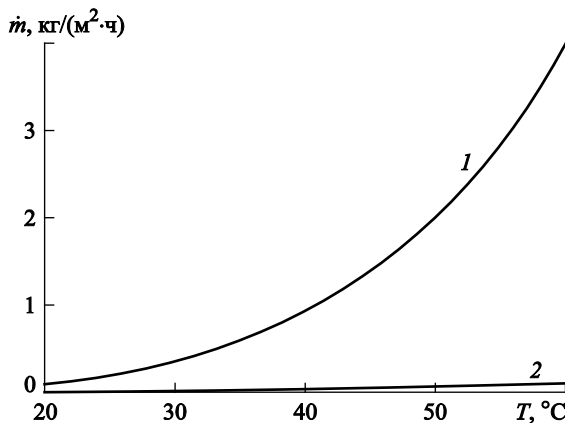
Рис. 6. Изменение в процессе нагрева плотности потока массы воды, испаряющейся с открытой поверхности резервуара (1) и при размещении на водной поверхности полых сферических изоляторов (2)
