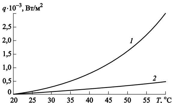
Рис. 3. Изменение плотности теплового потока с открытой поверхности (1) и средней плотности теплового потока через боковые поверхности и днище резервуара (2) в процессе нагрева
