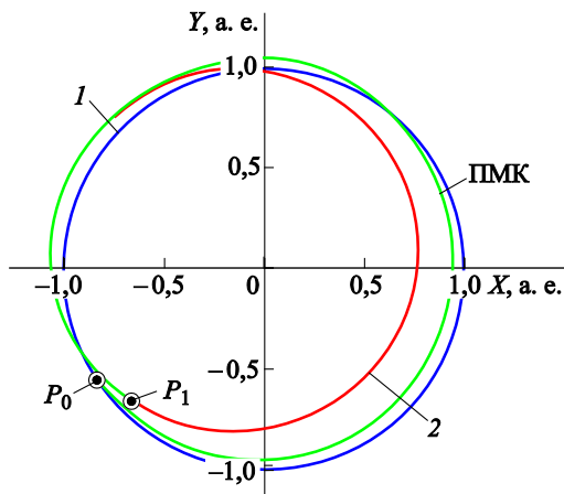
Рис. 2. Схема перелета ПМК с орбиты Земли (1) на орбиту Апофиса (2) (точки P_0 и P_1 соответствуют моментам отлета от Земли и подлета к астероиду)
