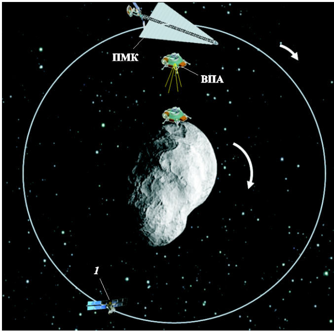
Рис. 4. Осуществление экспедиции на Апофис с установкой на синхронной экваториальной орбите ПМК над выбранной точкой посадки ВПА и спутника-ретронслятора (I). Стрелками обозначено направление вращения астероида вокруг своей оси и ПМК по орбите
