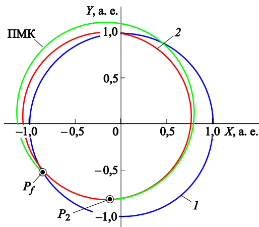
Рис. 3. Схема перелета ПМК с орбиты Апофиса (2) на орбиту Земли (1) (точки P_2 и P_f соответствуют моментам отлета от астероида и подлета к орбите Земли)
