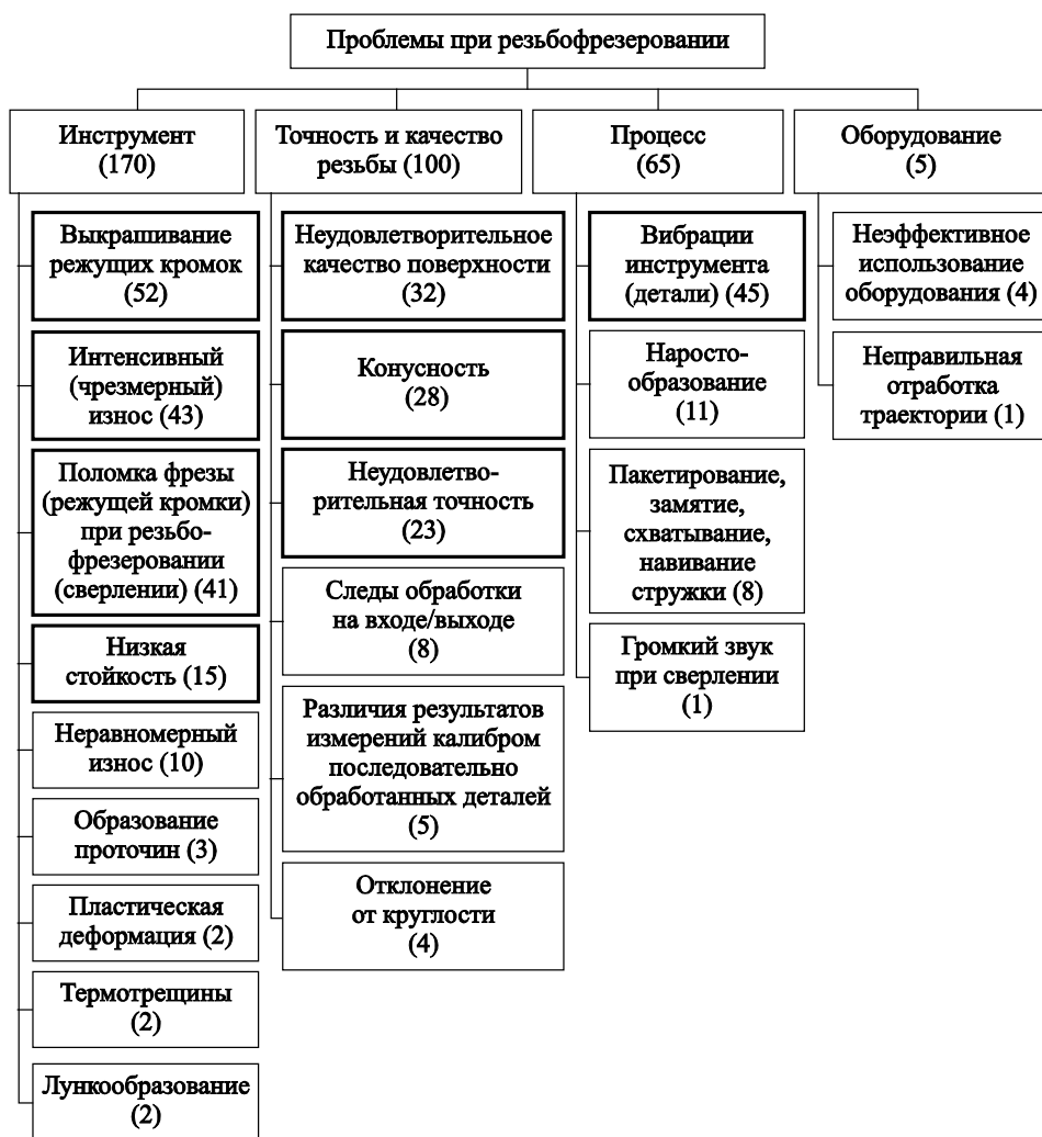
Рис. 3. Структура проблем при резбифрезеровании
