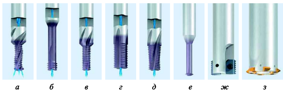
Рис. 2. Основные типы резбовых фрез
