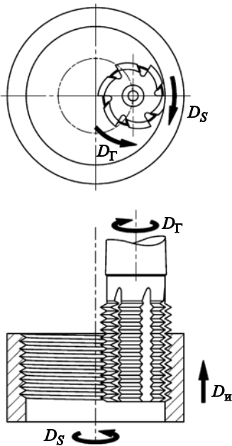
Рис. 1. Фрезерование внутренней резьбы гребенчатой концевой фрезой
