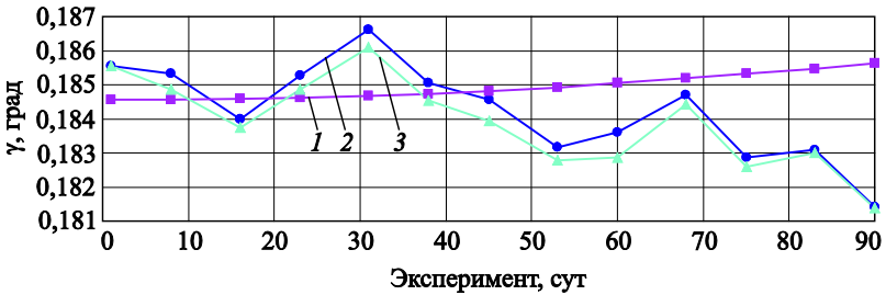
Рис. 10. Рассогласование по пространственному углу между орбитами: 1 — по начальному TLE; 2 — фактическое; 3 — по начальному ВС
