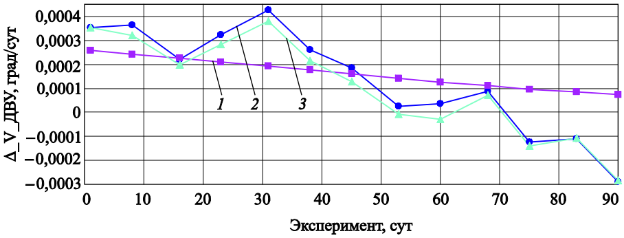
Рис. 8. Рассогласование по относительной скорости прецессии орбит: 1 — по начальному TLE; 2 — фактическое; 3 — по начальному ВС
