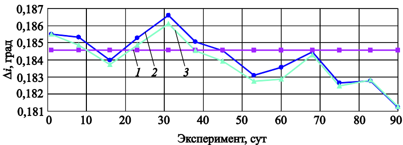
Рис. 11. Рассогласование наклонению орбит: 1 — по начальному TLE; 2 — фактическое; 3 — по начальному ВС
