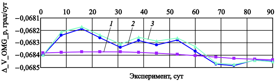
Рис. 9. Рассогласование по скорости поворота линии апсид: 1 — по начальному TLE; 2 — фактическое; 3 — по начальному ВС
