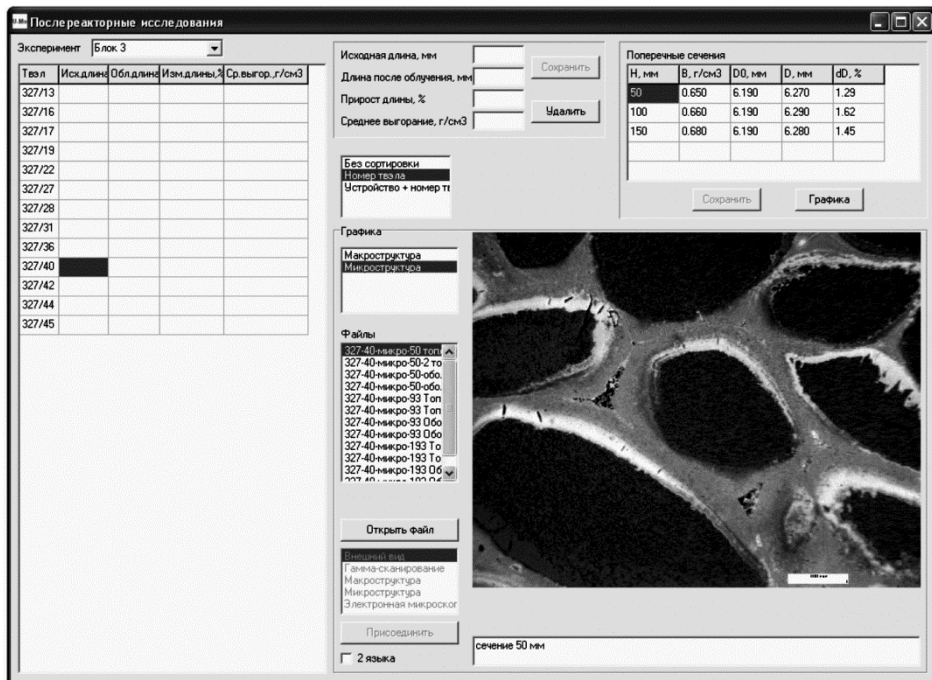
Рис. 3. Микроструктура поперечного сечения облученного ТВЭЛ с топливной композицией диоксид урана + алюминиевый сплав
