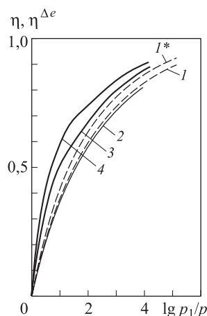
Рис. 1. Изменение термодинамического КПД в зависимости от отношения давления мгновенного взрыва к конечному давлению расширенных ПВ: I — расчет по (2) для \rho_0 = 0,88 \text{ г/см}^3 и \rho_0 = 1,5 \text{ г/см}^3 при \gamma = 1,24 ; I^* — расчет по (2) для \rho_0 = 0,88 \text{ г/см}^3 и \rho_0 = 1,5 \text{ г/см}^3 при \gamma = 1,28 ; 2 — \rho_0 = 0,88 \text{ г/см}^3 , e_1 = e_0 = 5,7 \text{ МДж/кг} , УРС — JWL; 3 — \rho_0 = 1,5 \text{ г/см}^3 , e_1 = e_0 = 5,7 \text{ МДж/кг} , УРС — JWL; 4 — \rho_0 = 1,5 \text{ г/см}^3 , e_1 = e_0 + \Delta e_{\text{EXP}}^C , \Delta e_{\text{EXP}}^C = 0,2 \text{ МДж/кг} , УРС — JWL
