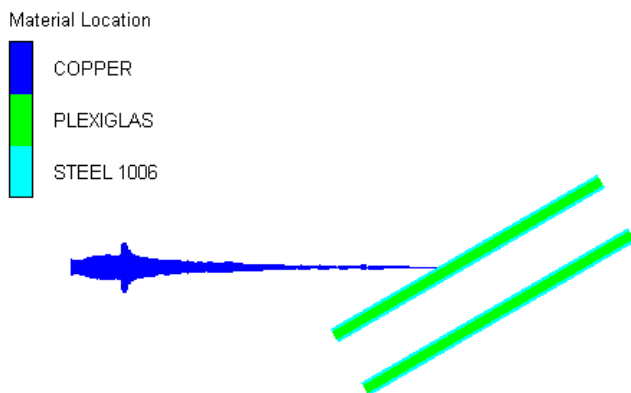
Рис. 4. Постановка задачи проникания КС через два параллельных невзрывных ЭДЗ
