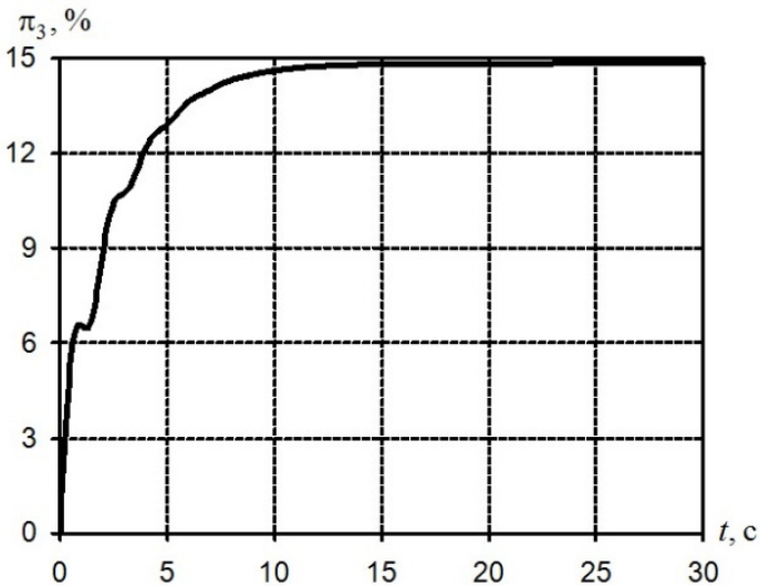
Рис. 2. Изменение давления \pi в производственном отборе турбины ПТ-25/30-90/10М с течением времени t
