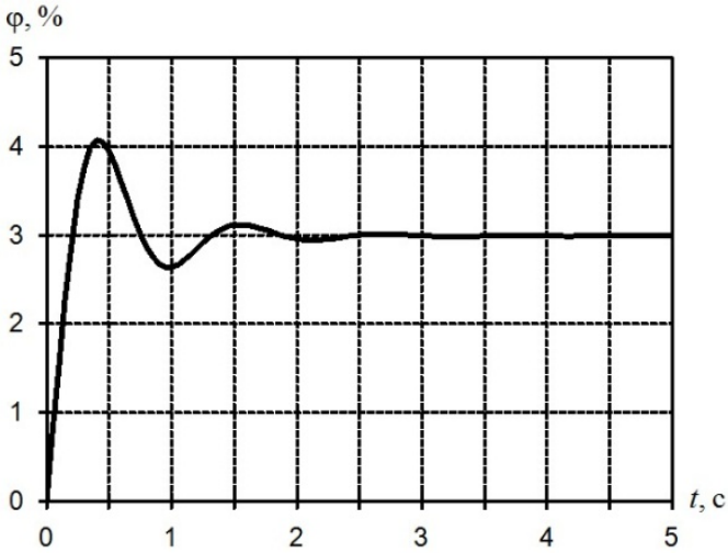
Рис. 1. Изменение частоты вращения \varphi турбины ПТ-25/30-90/10М с течением времени t
